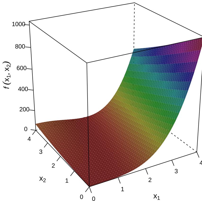
图 20.9: 类香蕉函数的曲面图
