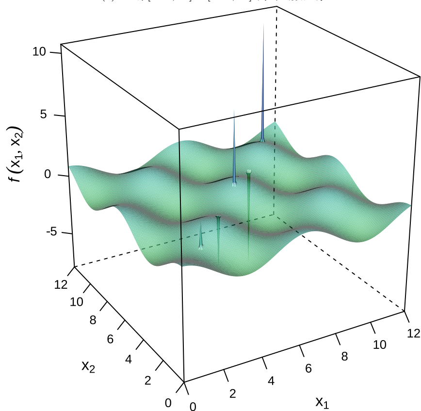
(b) 区域 [0, 12] \times [0, 12] 内的函数图像
