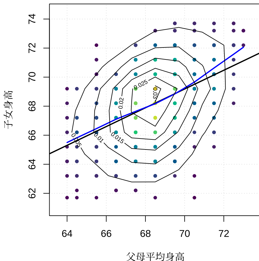
图 13.3: 二维核密度估计与二元正态分布
