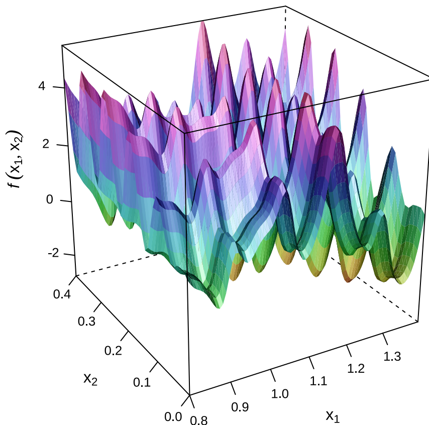
图 20.10: 目标函数的曲面图
