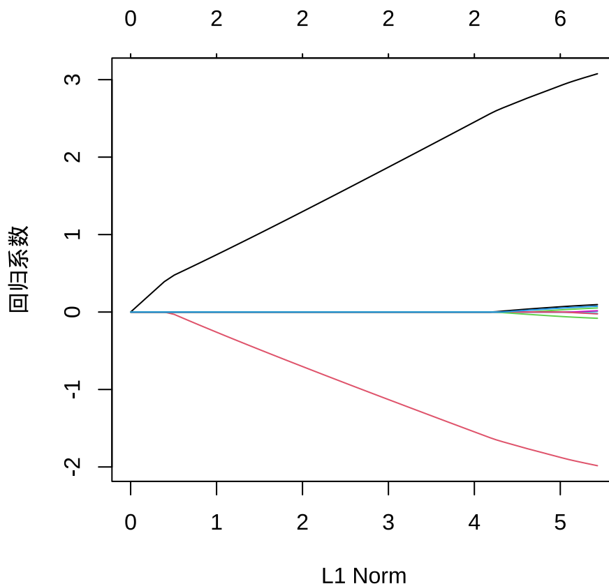
图 19.3: 回归系数的迭代路径
