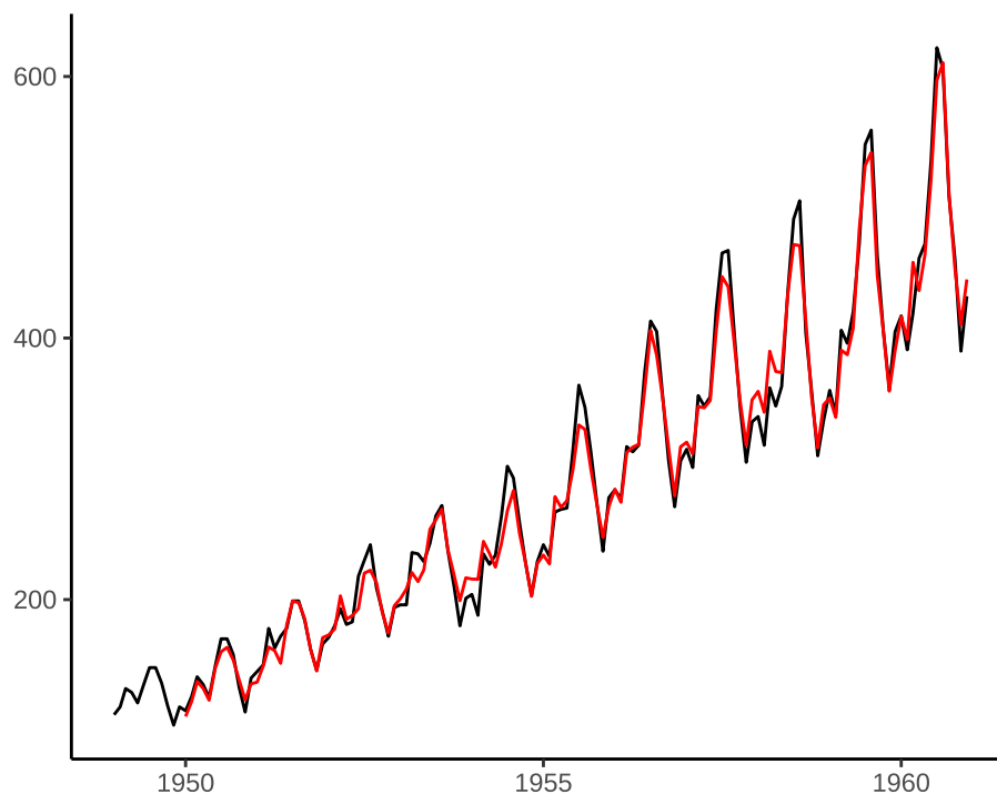
图 18.12: 可加 Holt-Winters 平滑模型拟合
