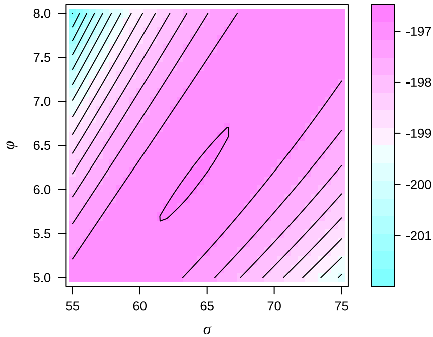
图 21.4: 对数似然函数的等高线图
