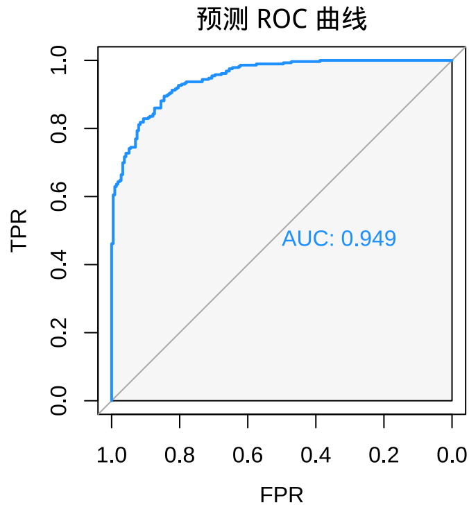
图 19.5: ROC 曲线
