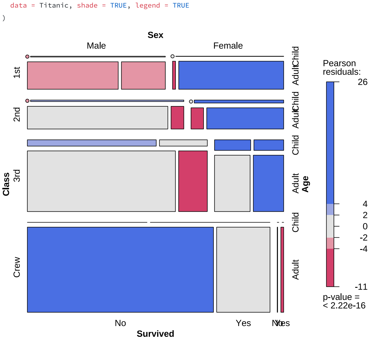
图 14.4: 马赛克图展示多维分类数据
