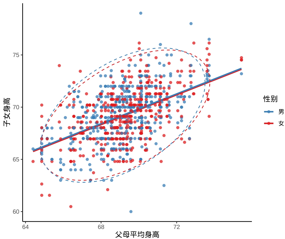
图 13.2: 子代身高与亲代身高的关系
