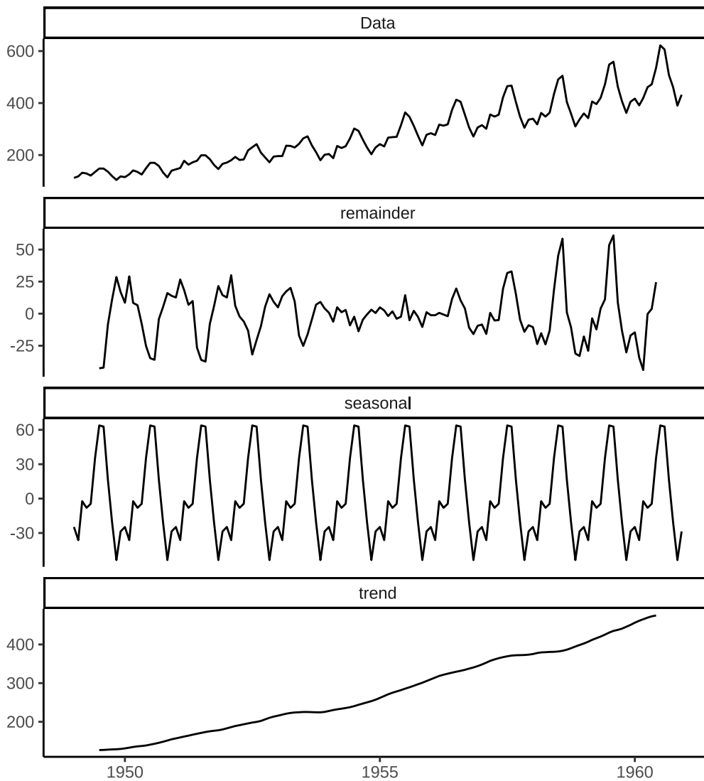
图 18.14: 变化趋势的分解
