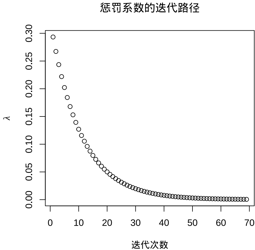
图 19.4: 惩罚系数的迭代路径
