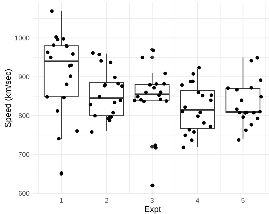
图 12.8: 1879 年迈克尔逊光速实验数据
