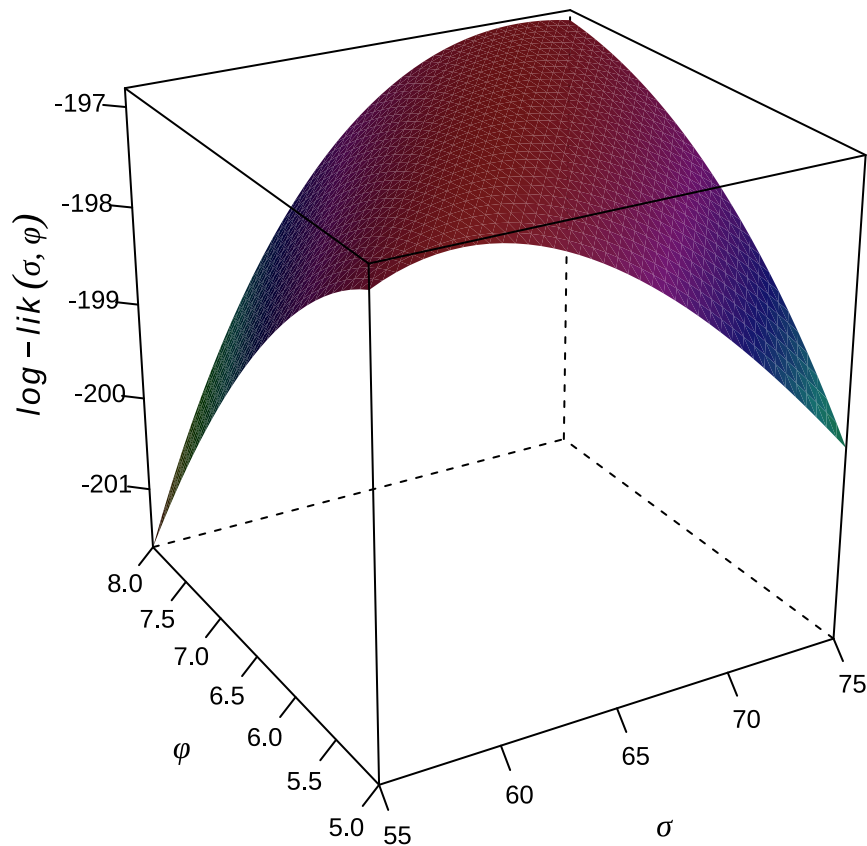
图 21.3: 对数似然函数的曲面图
