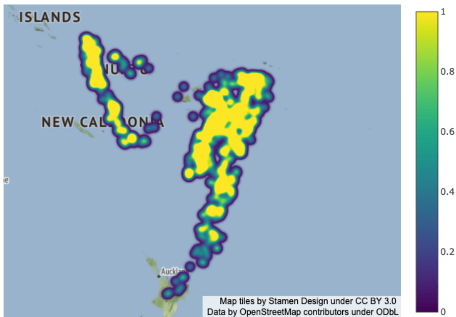
图 6.6: 空间点数据的核密度估计
