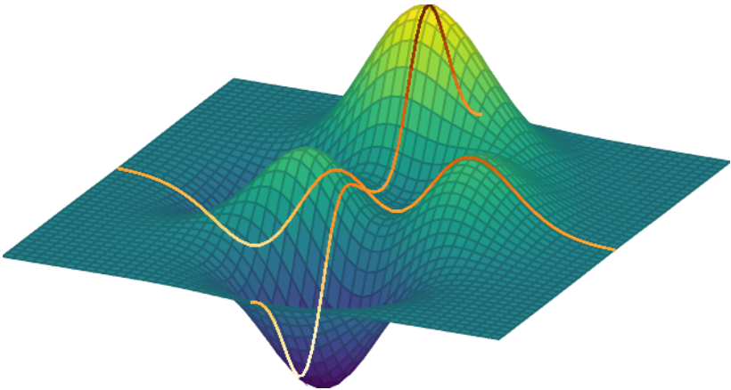
图 10.5: Peaks 函数图像
