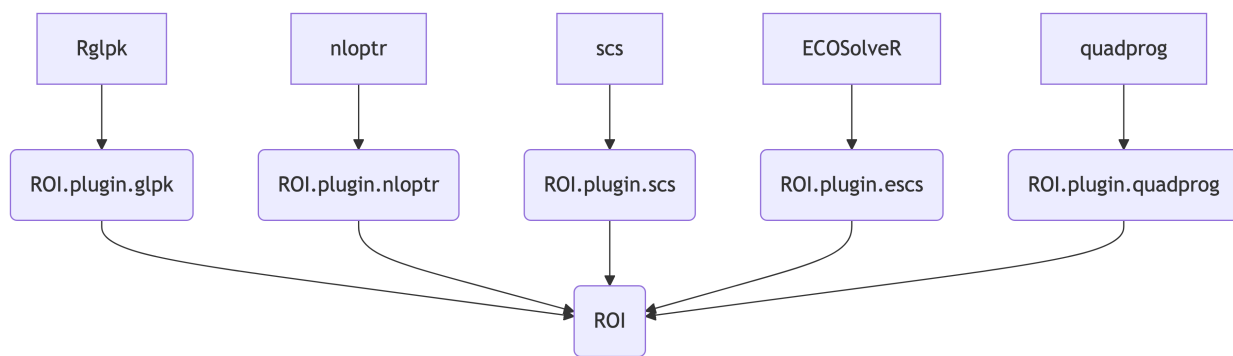
图 20.1: 数值优化扩展包、插件包和 ROI 包的关系图
