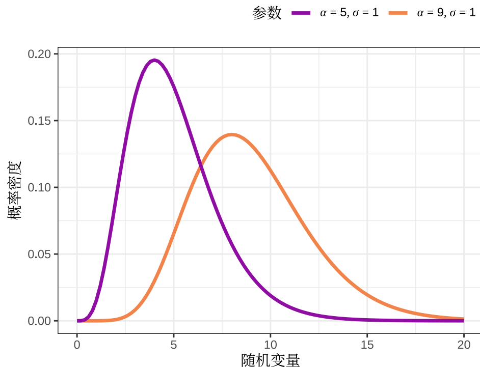
图 21.5: 伽马分布的概率密度函数
