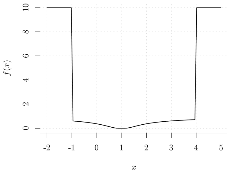
图 20.5: 一维函数图像
