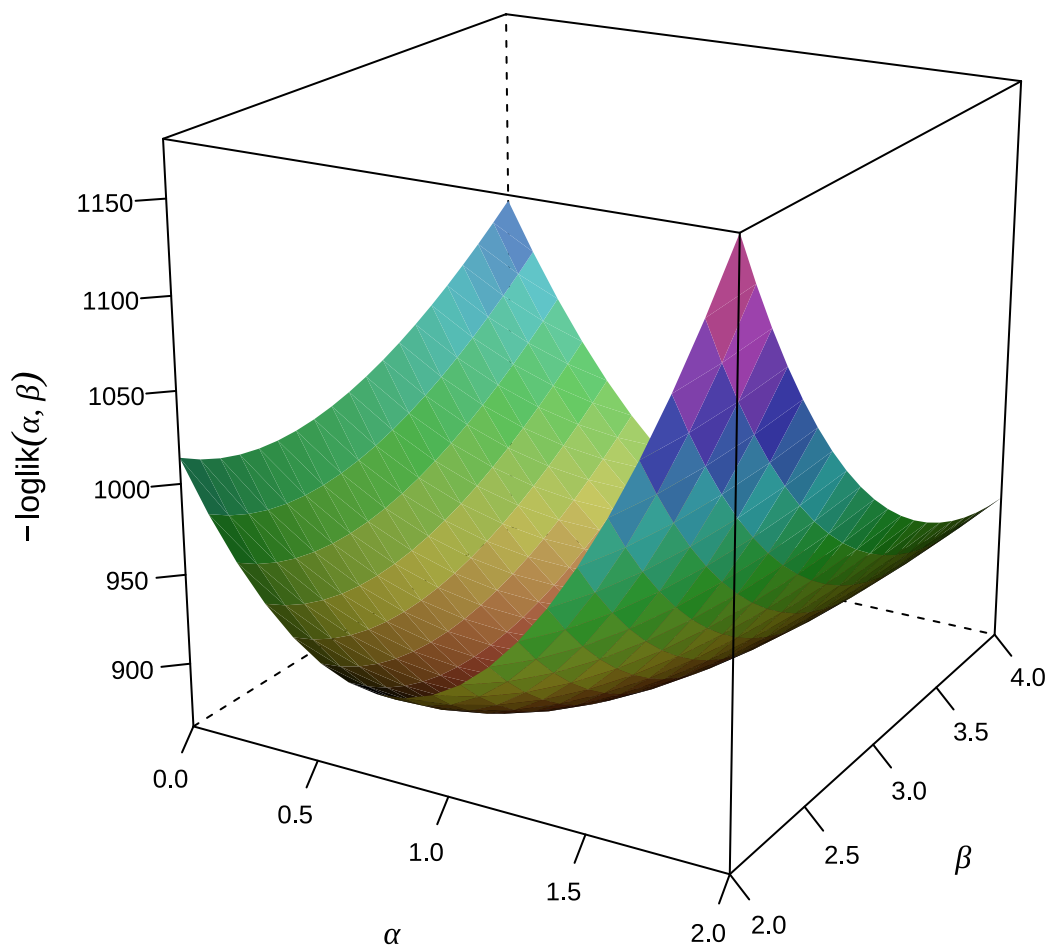
图 19.2: 二维情形下的逻辑回归模型的负对数似然函数曲面
