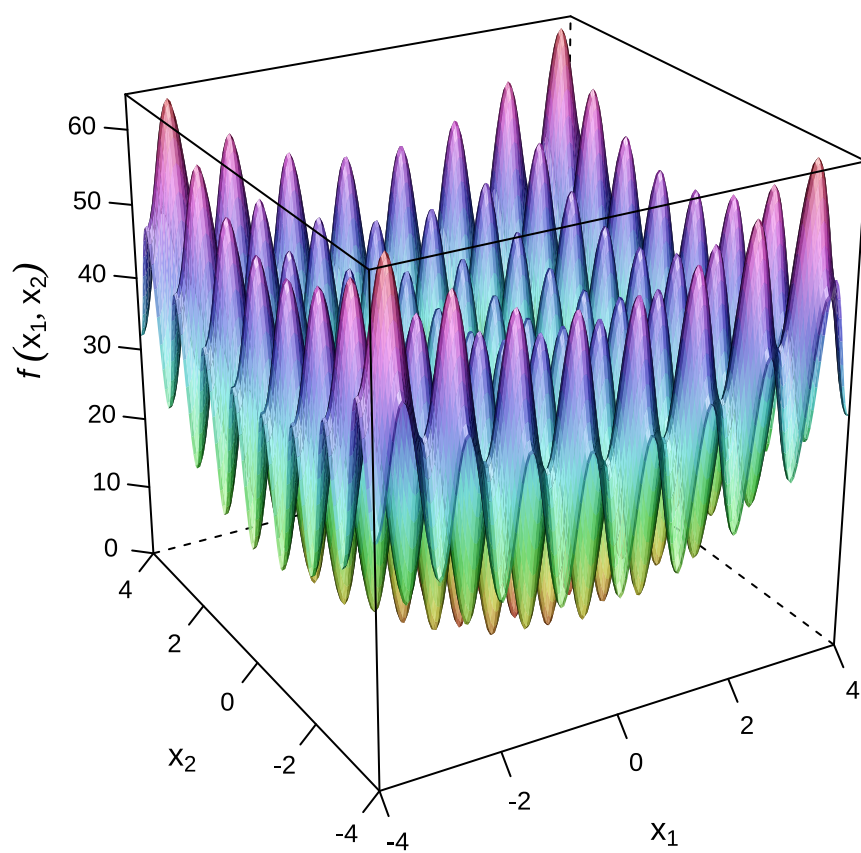
图 20.7: 二维 Rastrigin 函数图像
